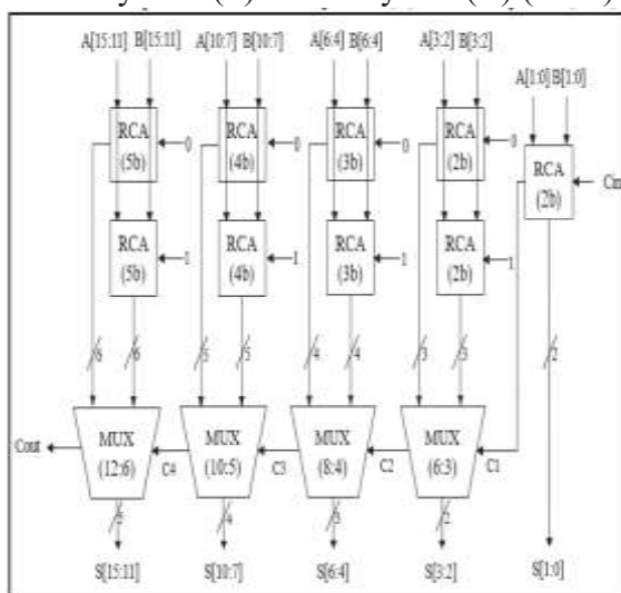
Fig. 3. 16-bit SRCSA
